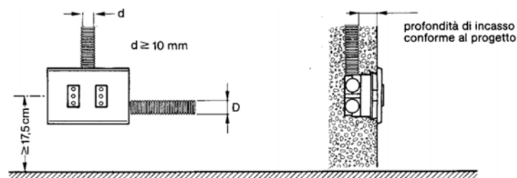
Figura 15.1 Criteri di installazione degli impianti incassati e similari
