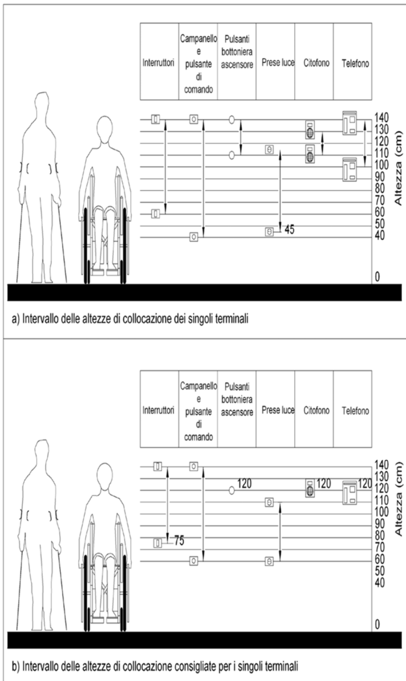
Figura 15.2 Altezze consigliate per i terminali degli impianti elettrici e telefonici
